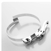
Car-Grip Snabbklämma Specialklämma för montering av Carflex Super- och Master-PUR STEP-slangar på mobila och stationära installationer
